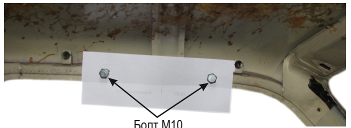
Рис.3 Установка шаблонов. Вид изнутри автомобиля
